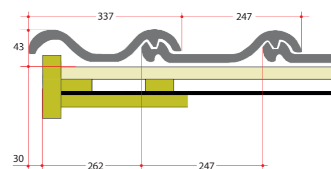
Ortgangausbildung mit Doppelkremper und Ortgangbrett
