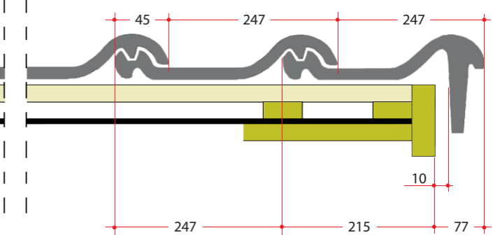
Detail van dubbel welpan met overstek en windveer
