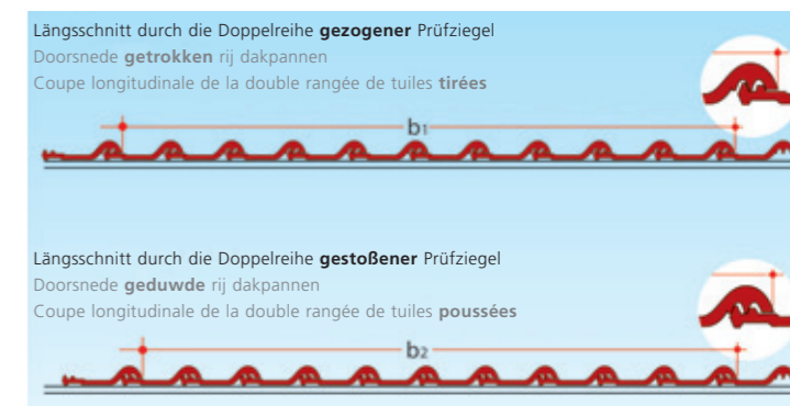
Orientierungs-Deckbreiten (cm) nach Anzahl der Ziegelreihen ohne GOZ oder Doppelkremper Dekbreedte (cm) met he aantal rijen dakpannen (ter orientatie)
