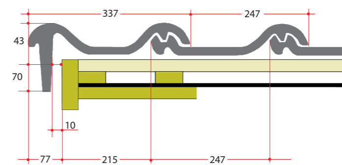
Ortgangausbildung mit Doppelkremper und Ortgangbrett
