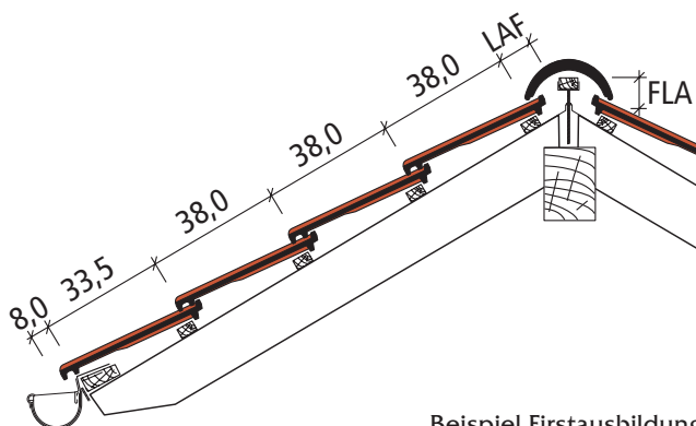
Beispiel Firstausbildung
